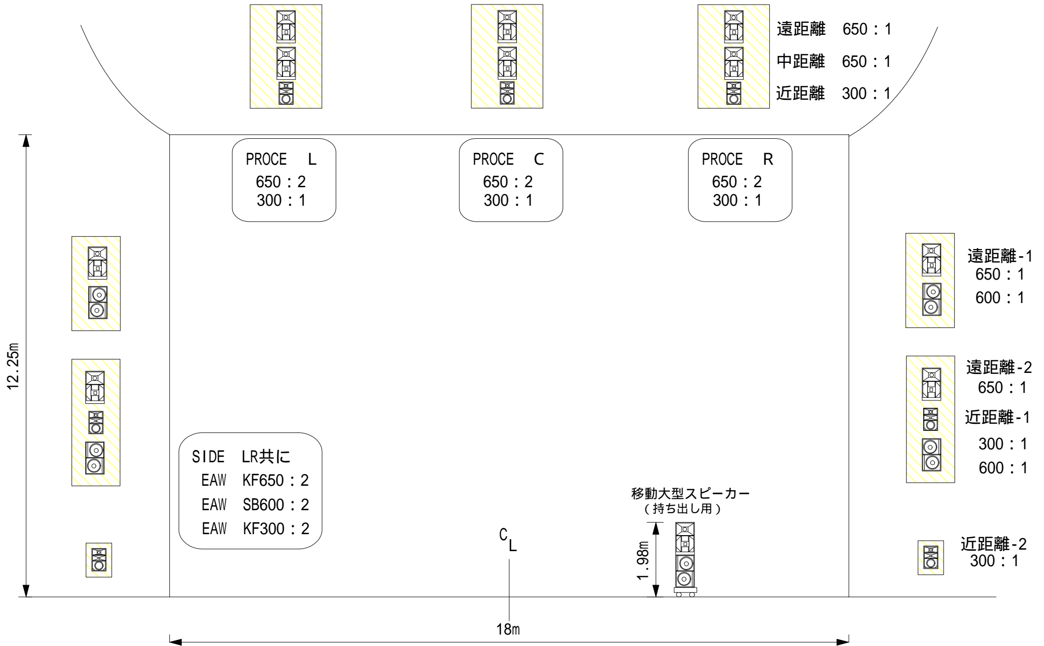
びわ湖ホール 大ホール プロセニアムサイドスピーカー配置図
